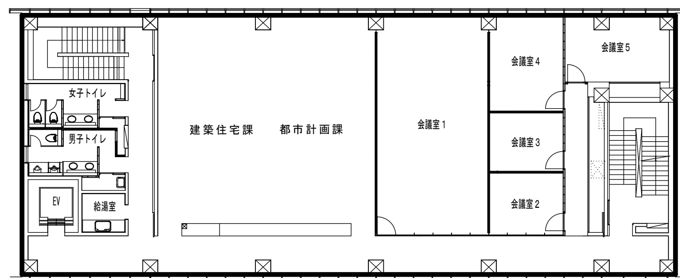
秩父市歴史文化伝承館 5階配置図
