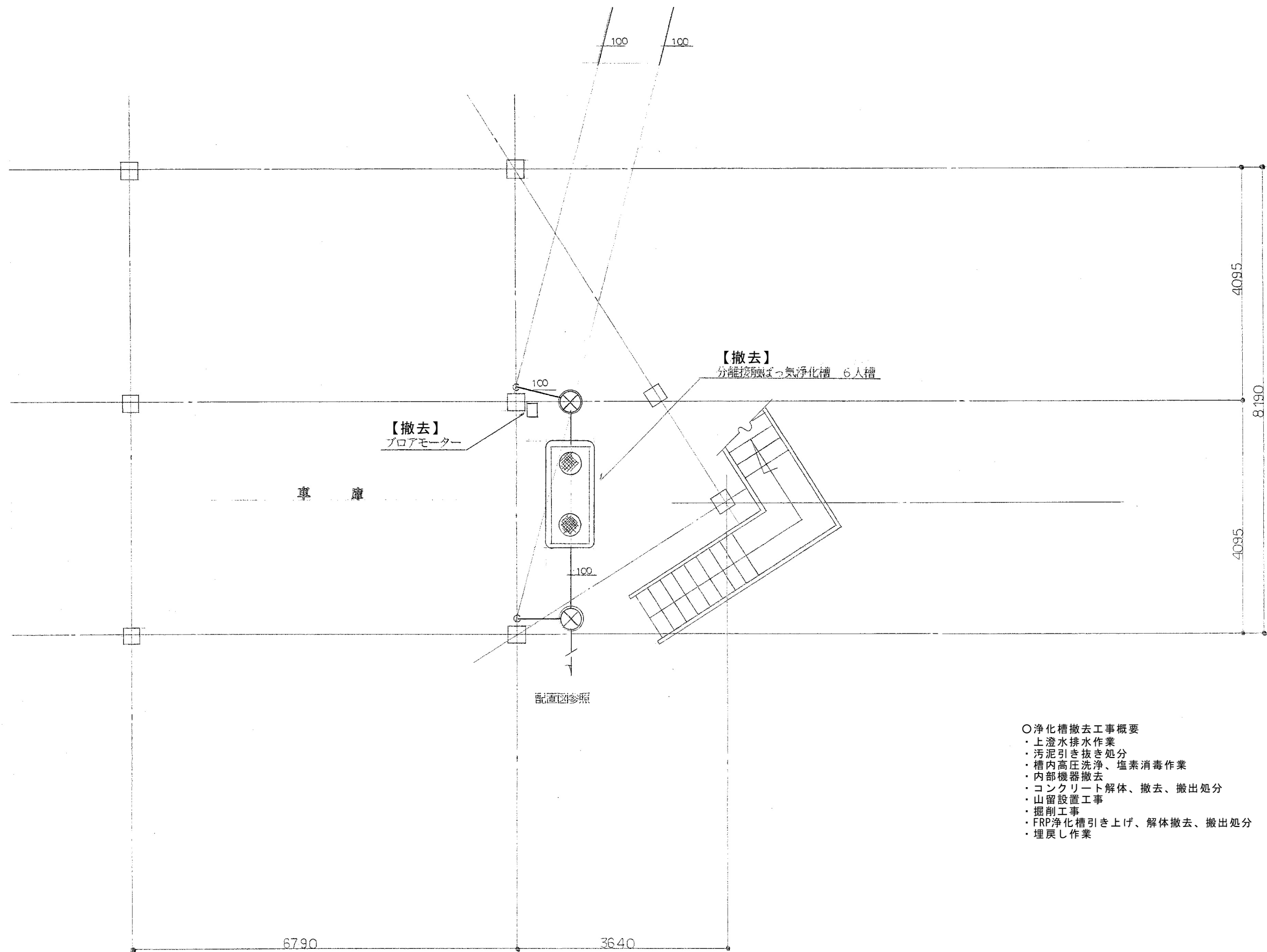
し尿浄化槽設備図 S=1/50
